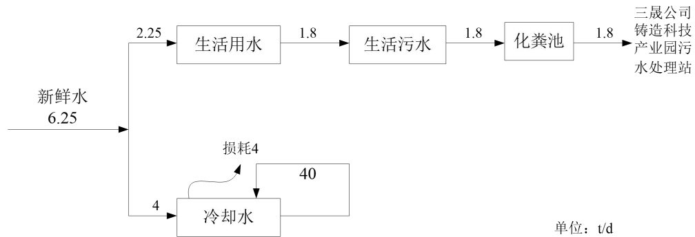
图 2.7-1 项目水平衡图
