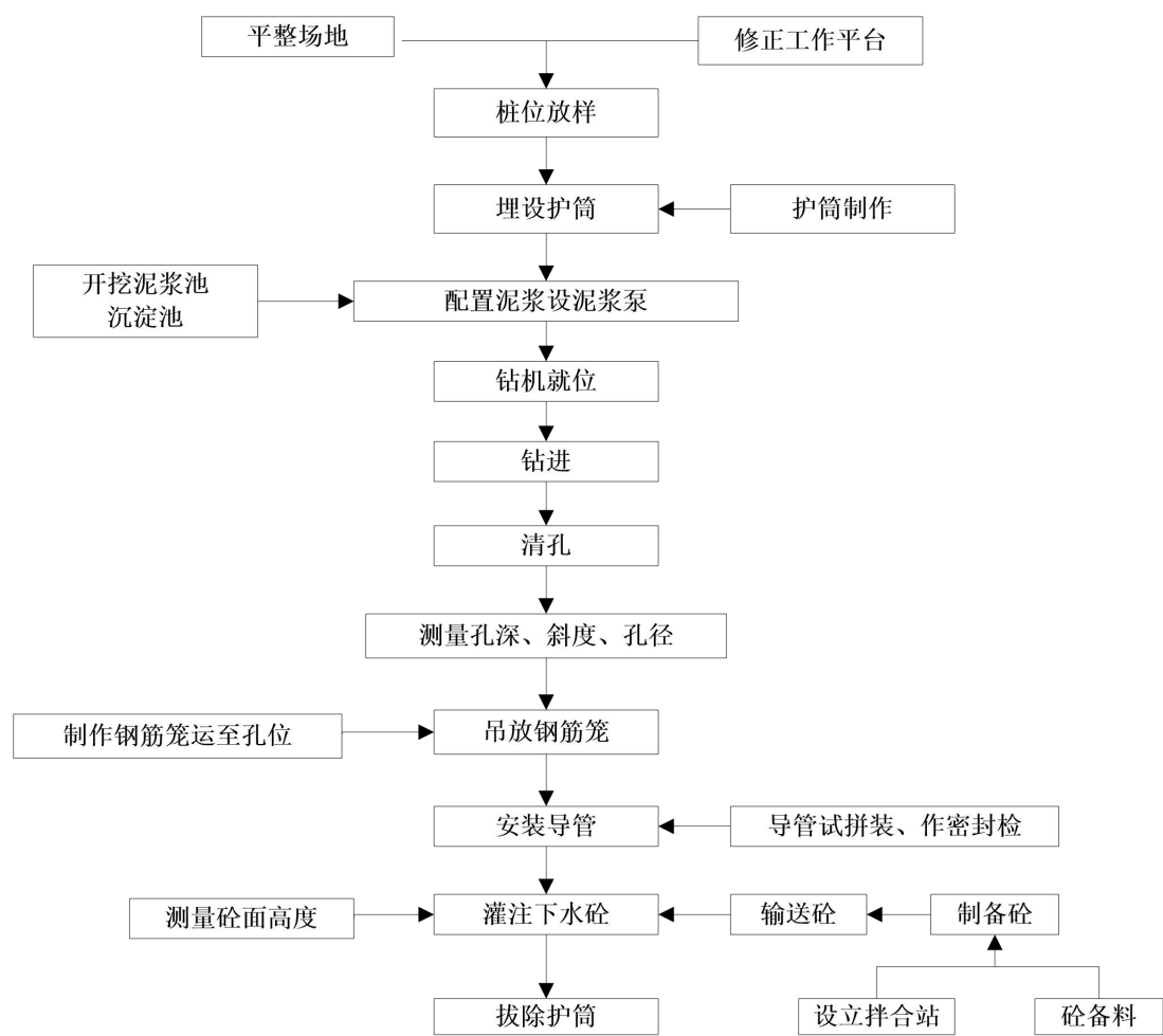
图 2.9-4 桥梁钻孔灌注桩施工工艺流程
