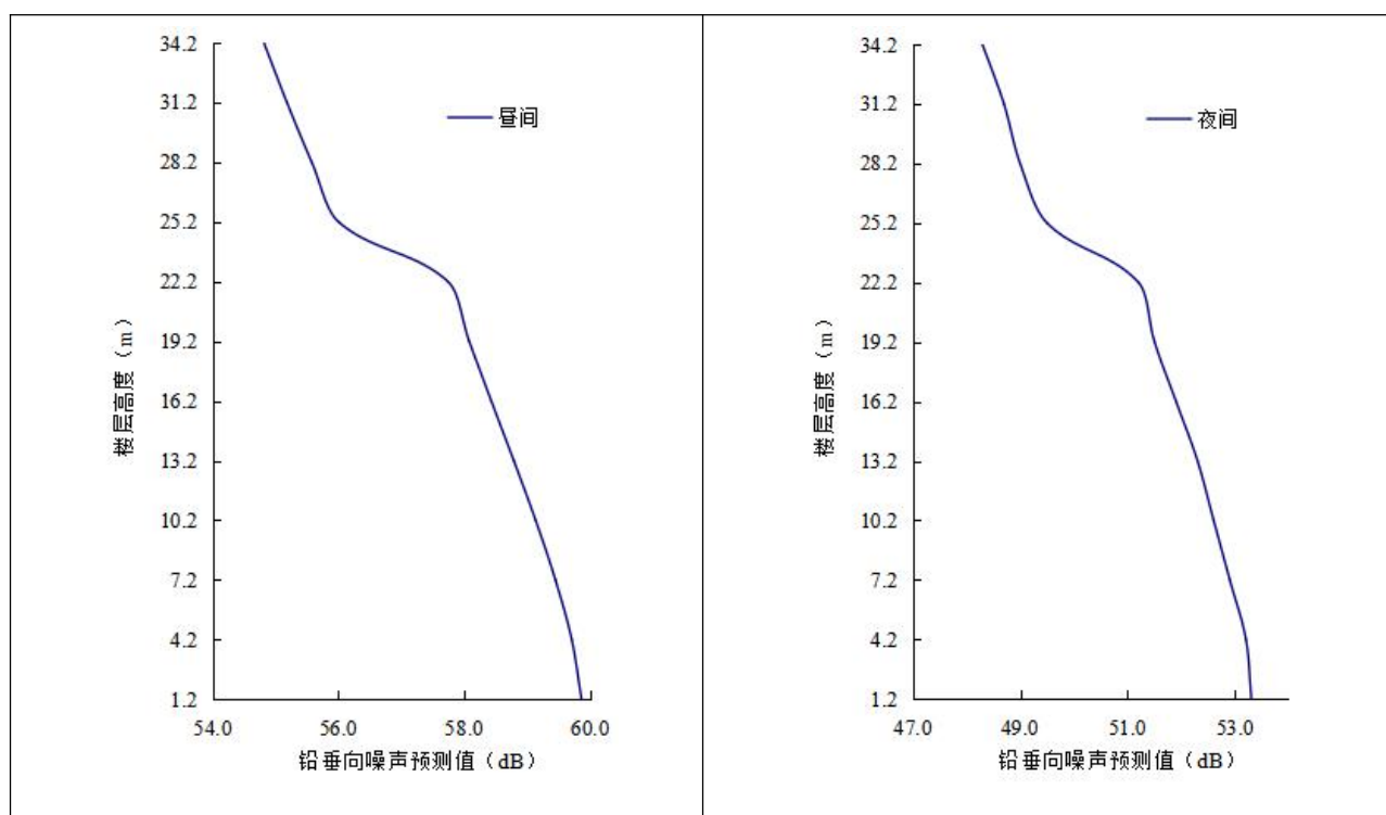
图 4.2-10 营运中期交通噪声铅垂向分布图
