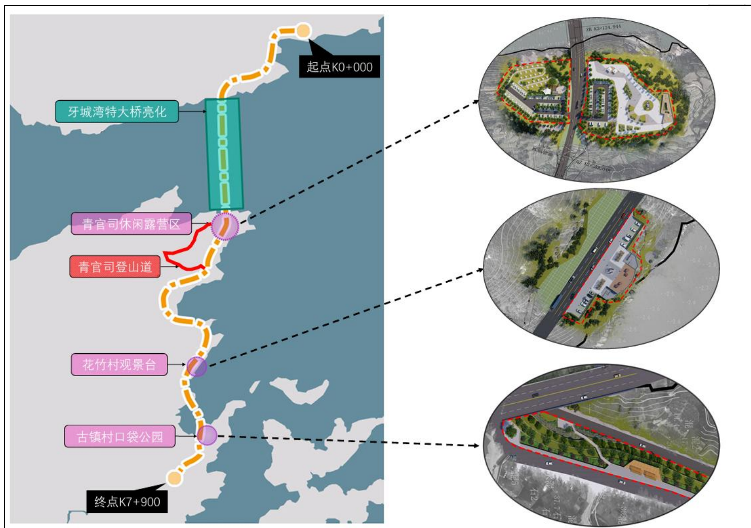
图 2.4-20 风景道工程位置图
