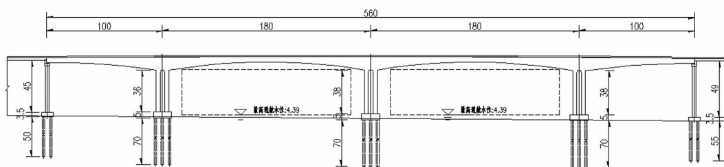
图 2.4-6 2×180m 连续钢构方案立面布置图 (单位: m)
