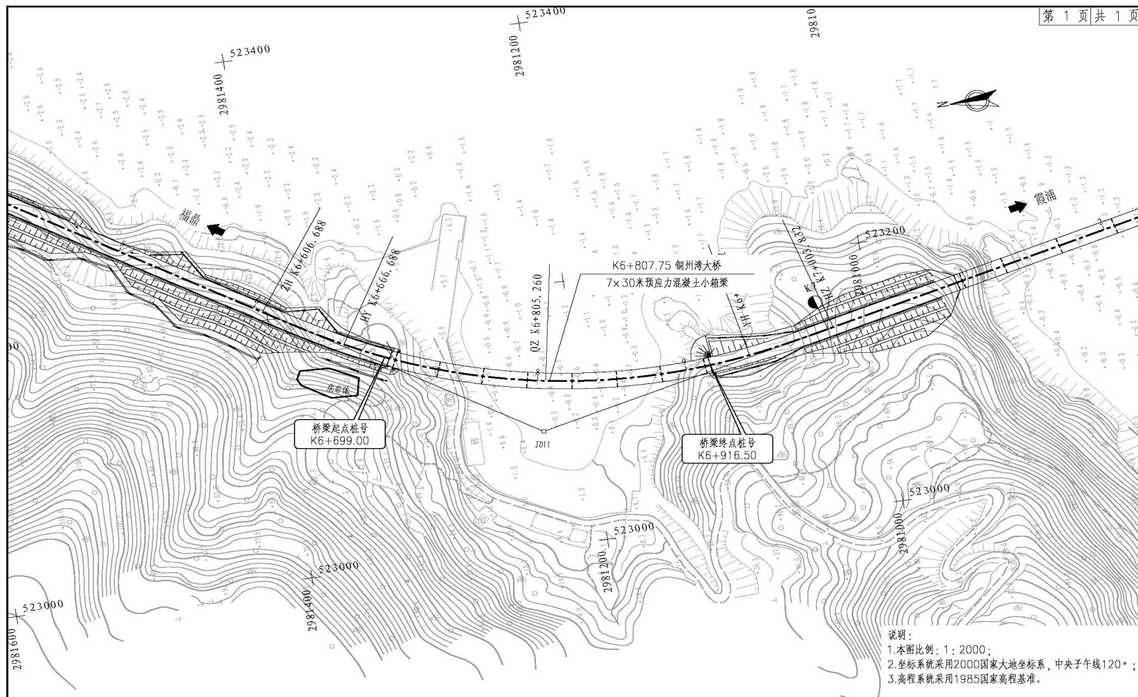
图 2.4-15 铜洲湾大桥桥位平面图
