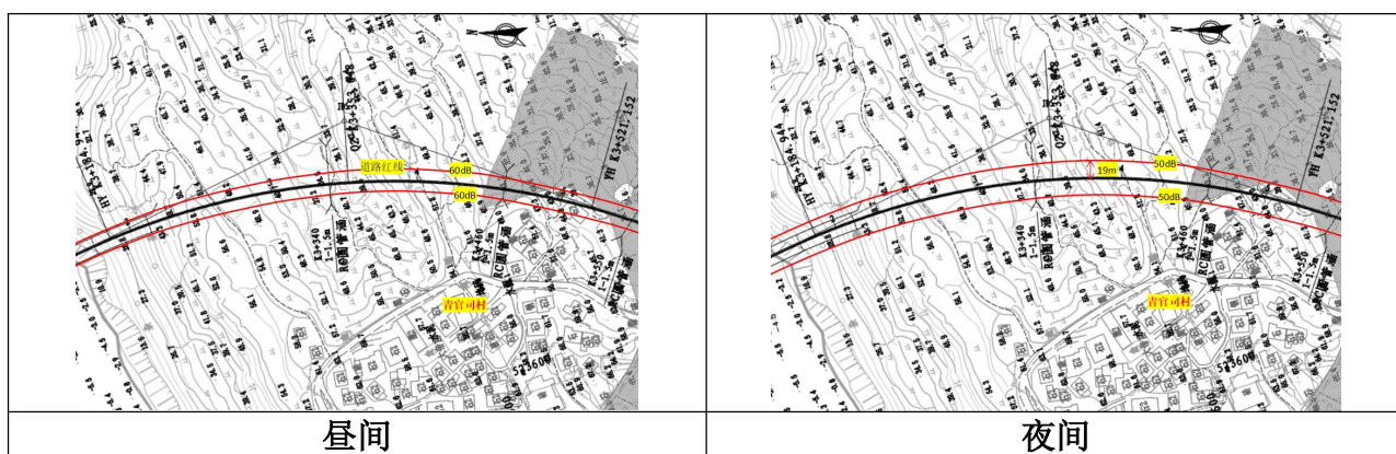
图 4.2-8 中期交通噪声等声值线图
