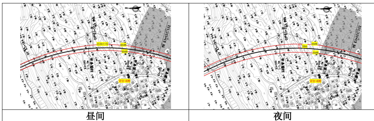
图 4.2-7 近期交通噪声等声值线图
