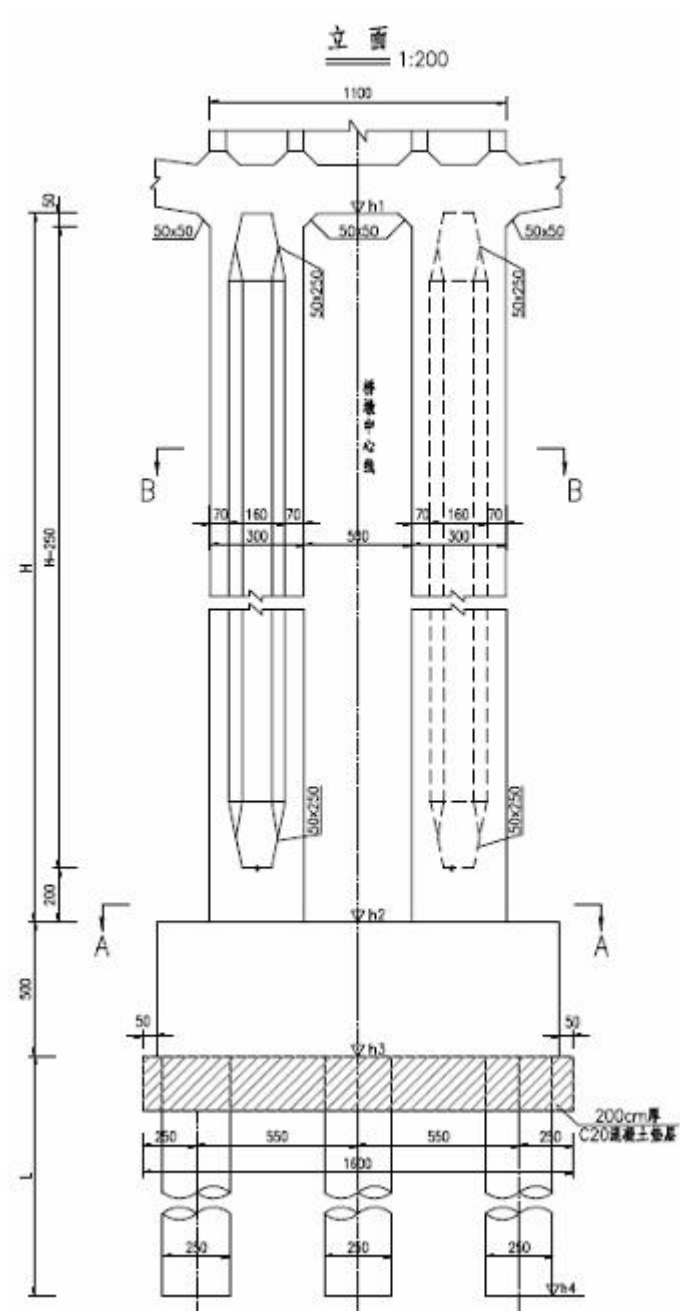
图 2.4-8 下部结构一般构造 (单位: cm)
