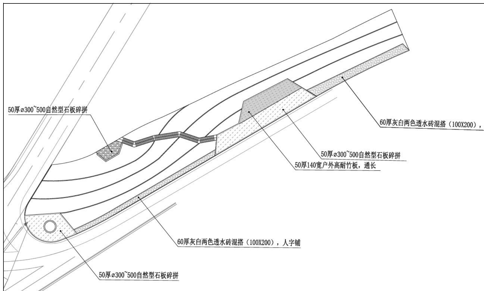
图 2.4-19 古镇口袋公园布置图
