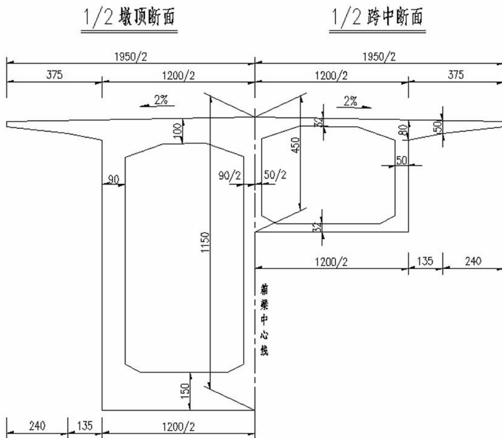
图 2.4-7 主梁典型断面（单位：cm）
