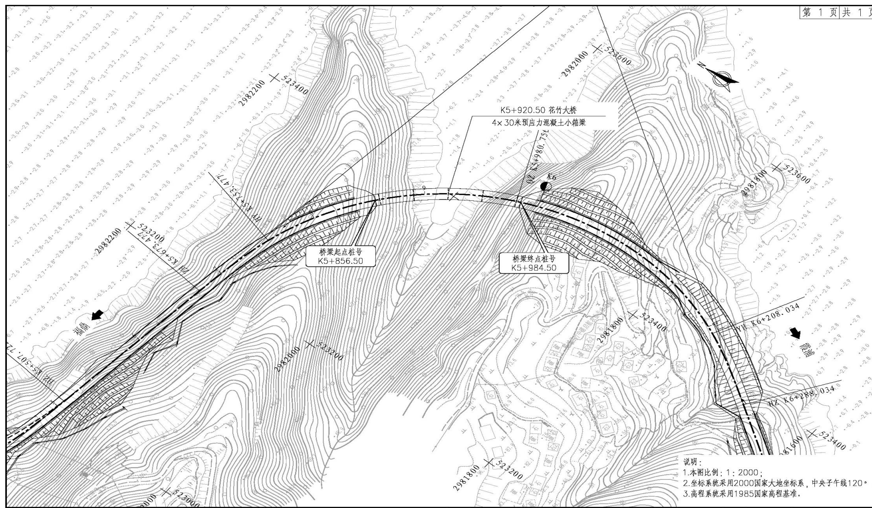
图 2.4-14 花竹大桥桥位平面图
