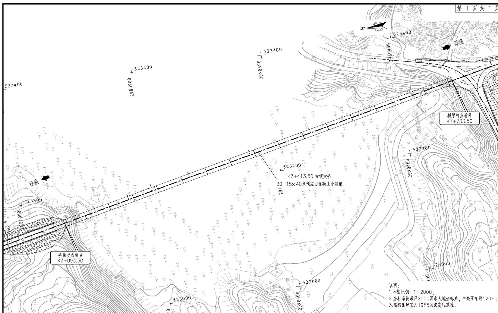
图 2.4-16 古镇大桥桥位平面图
