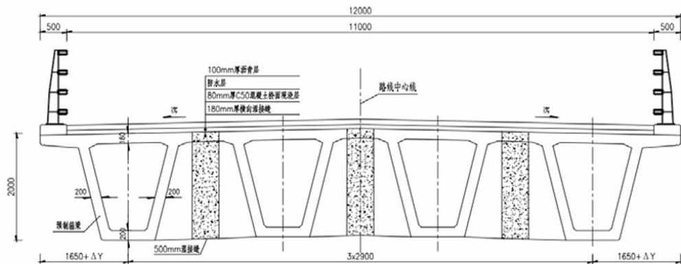
图 2.4-3 12m 宽桥梁标准横断面（单位：mm）
