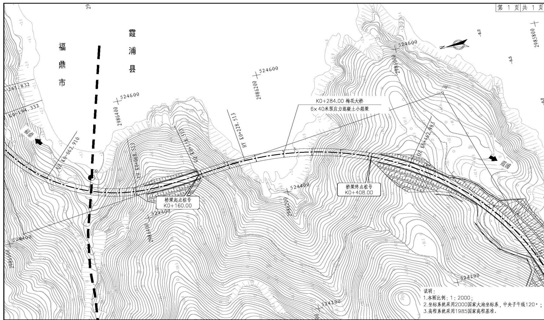
图 2.4-12 梅花大桥桥位平面图
