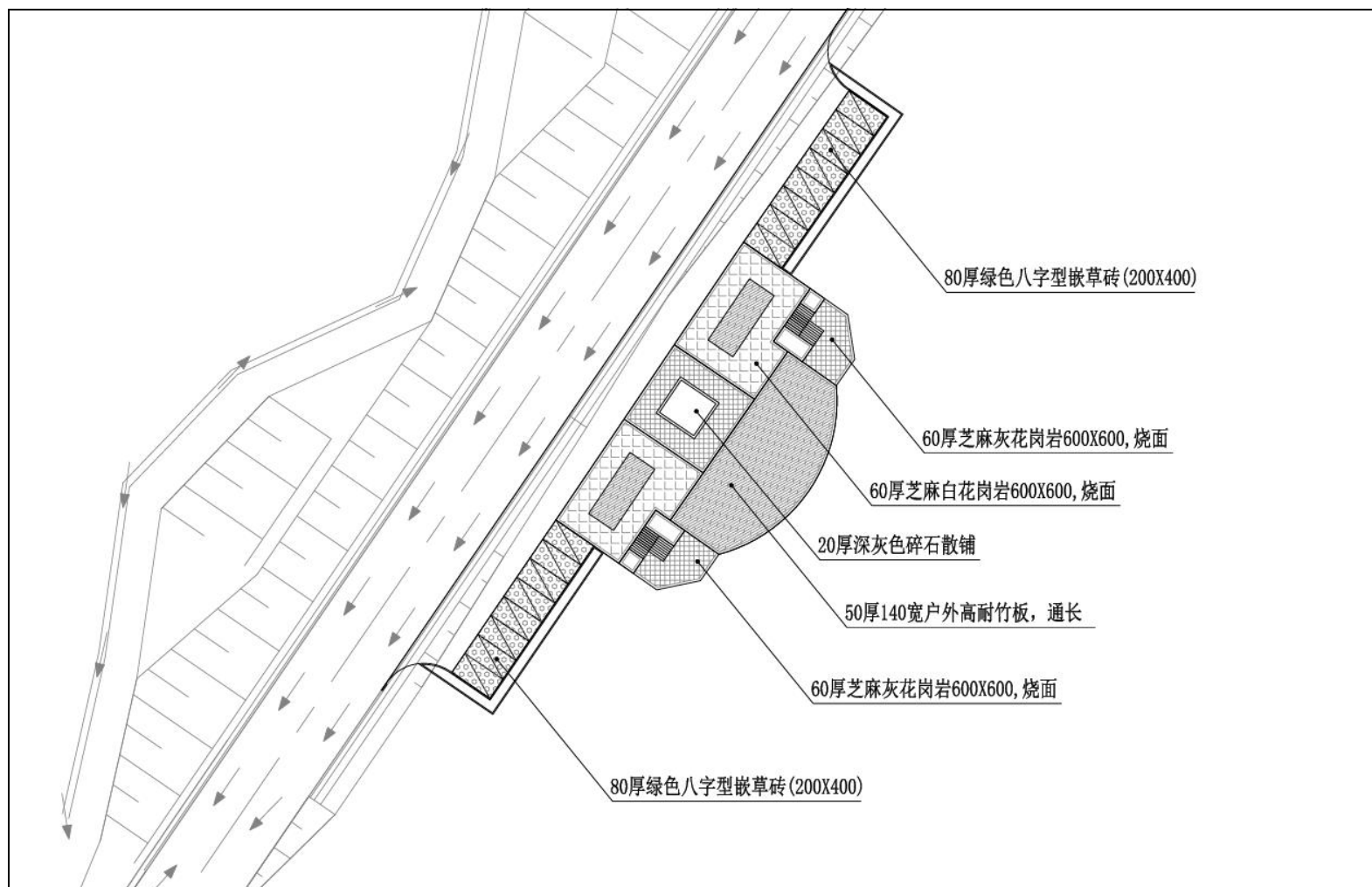
图 2.4-18 花竹村观景台平面图
