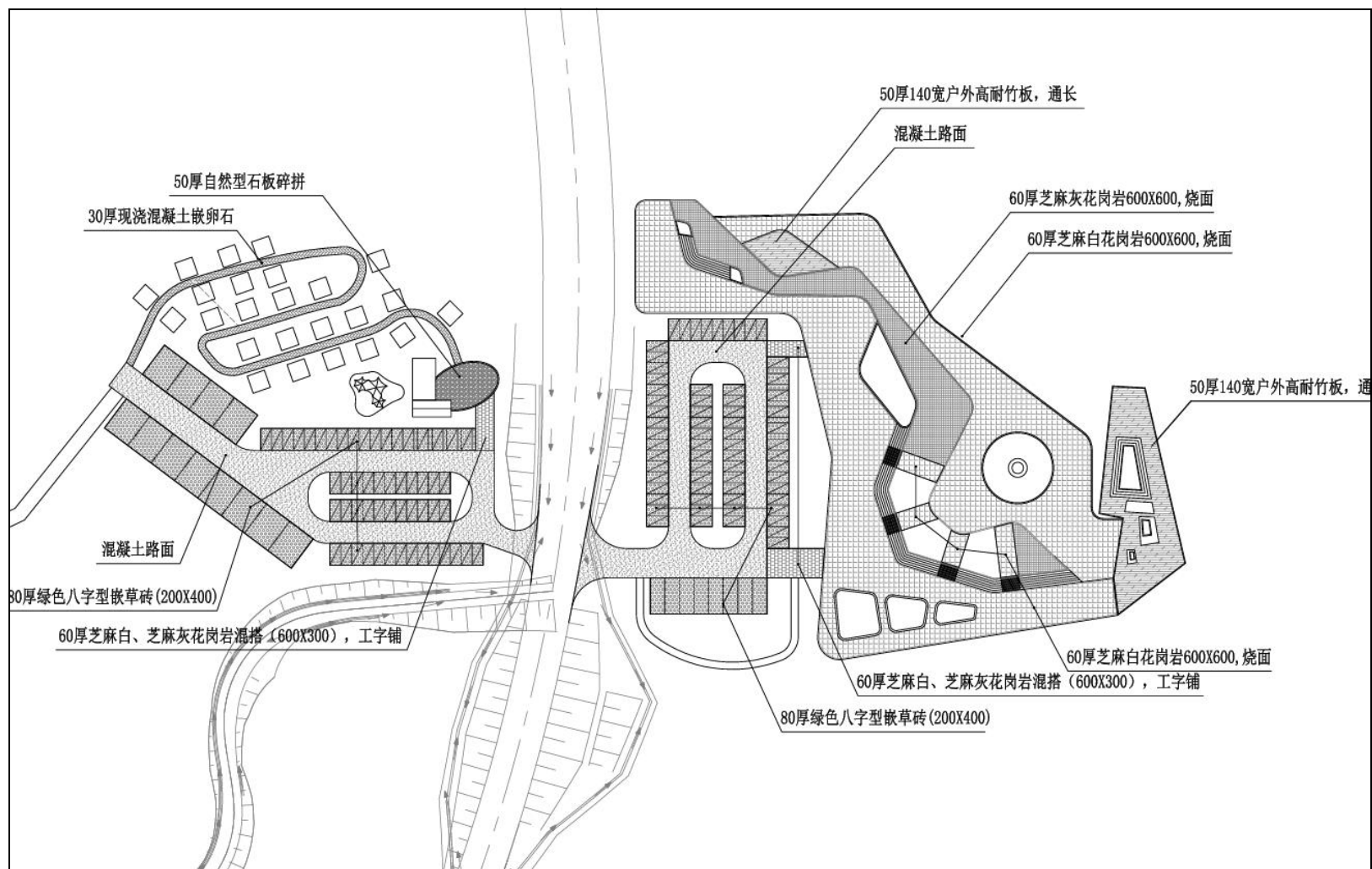
图 2.4-17 青官司休闲露营区布置图
