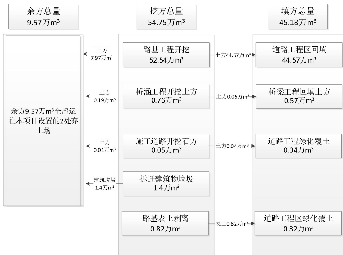
图 2.5-1 工程土石方平衡图(单位: 万 m³)
