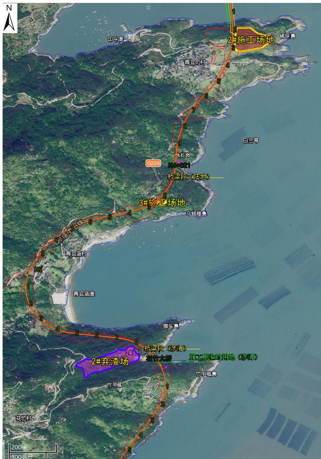
图 2.9-1 施工三场位置示意图（2）
