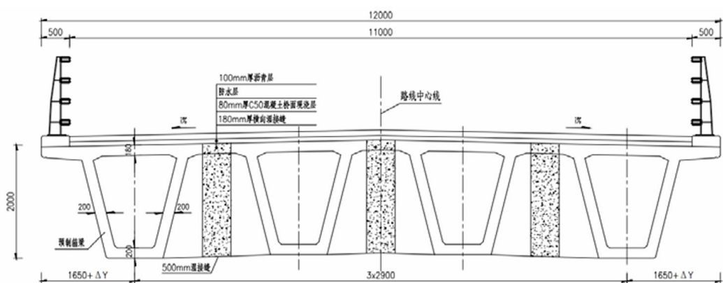
图 2.4-5 12m 宽桥梁标准横断面
