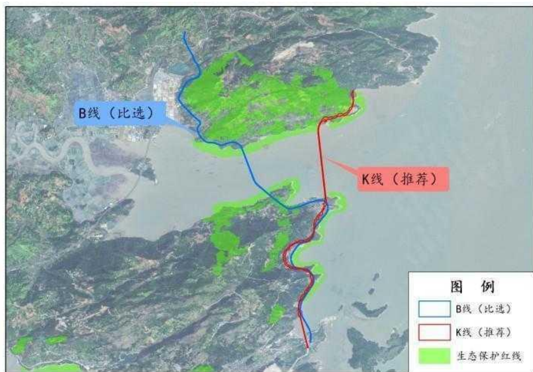
图2.10-6 线路对比方案
