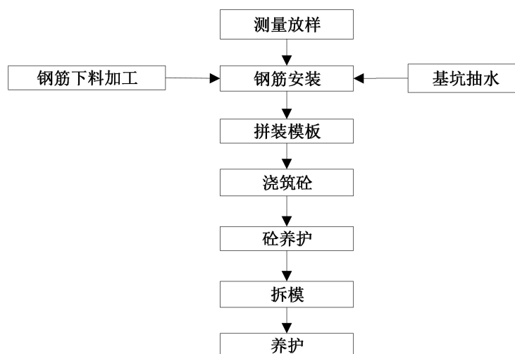
图 2.9-5 桥墩桥台施工工艺流程
