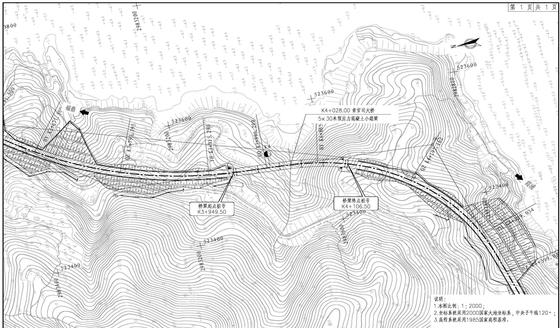
图 2.4-13 青官司大桥桥位平面图
