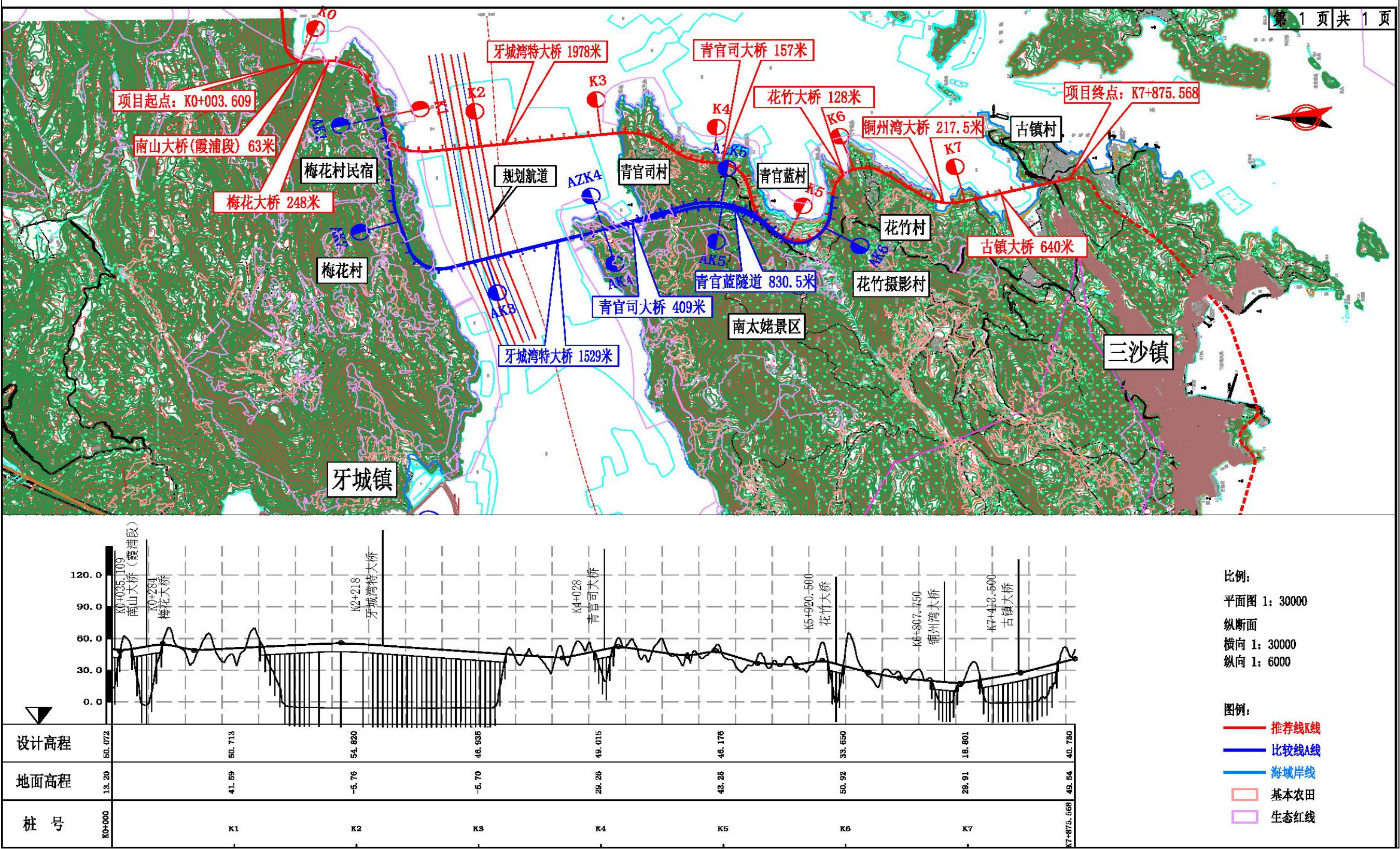
图 2.1-2 本项目起点终点平面布置图
